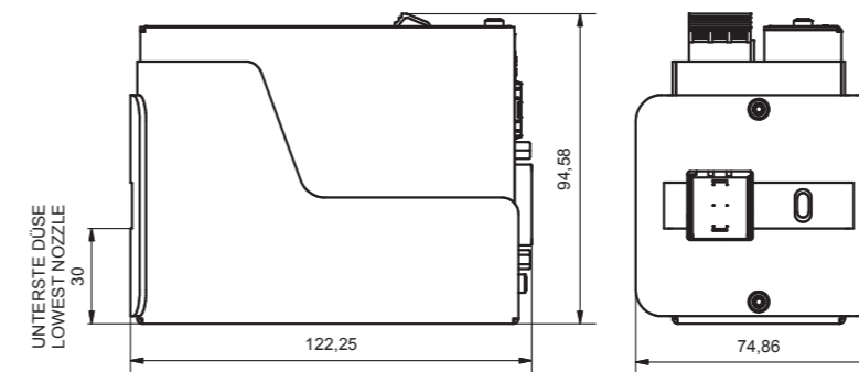
Technische Maßzeichnung
